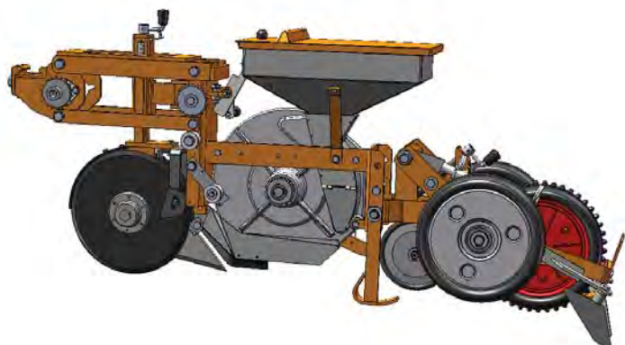
Mulch- und Direktsaatausrüstung mit PUMA-Rollen
