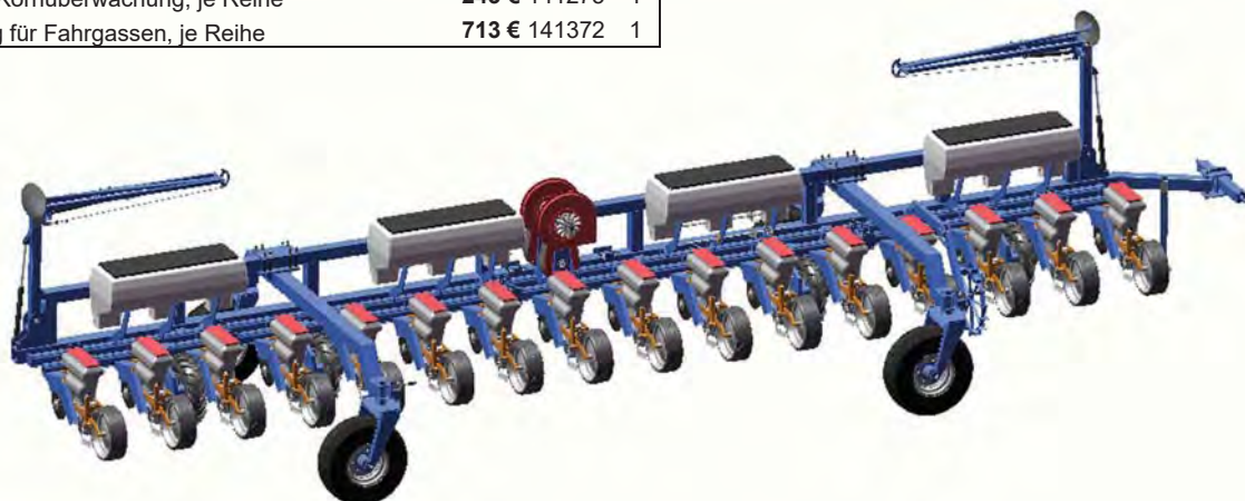
P4000 - 16 x 70 cm für Mais mit Düngerstreuer und Scheibendüngerscharen
