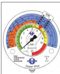
Mechanische Armatur Handbedienung
