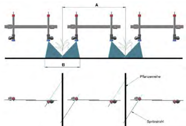
Bandspritze unter die Blätter
