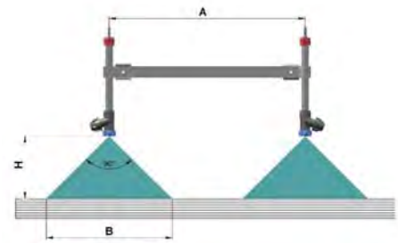
Bandspritze direkt auf die Pflanze
