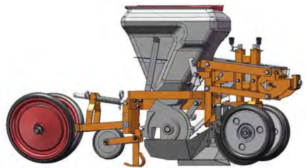
P4000 mit Schneidscheiben und großer Andruckrolle 500 mm
