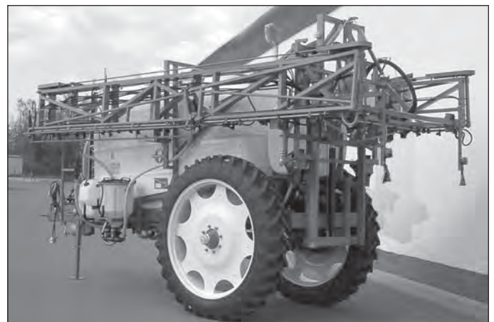
ASP 5 600 I mit Spritzrahmen 30 m Seitenklappung
